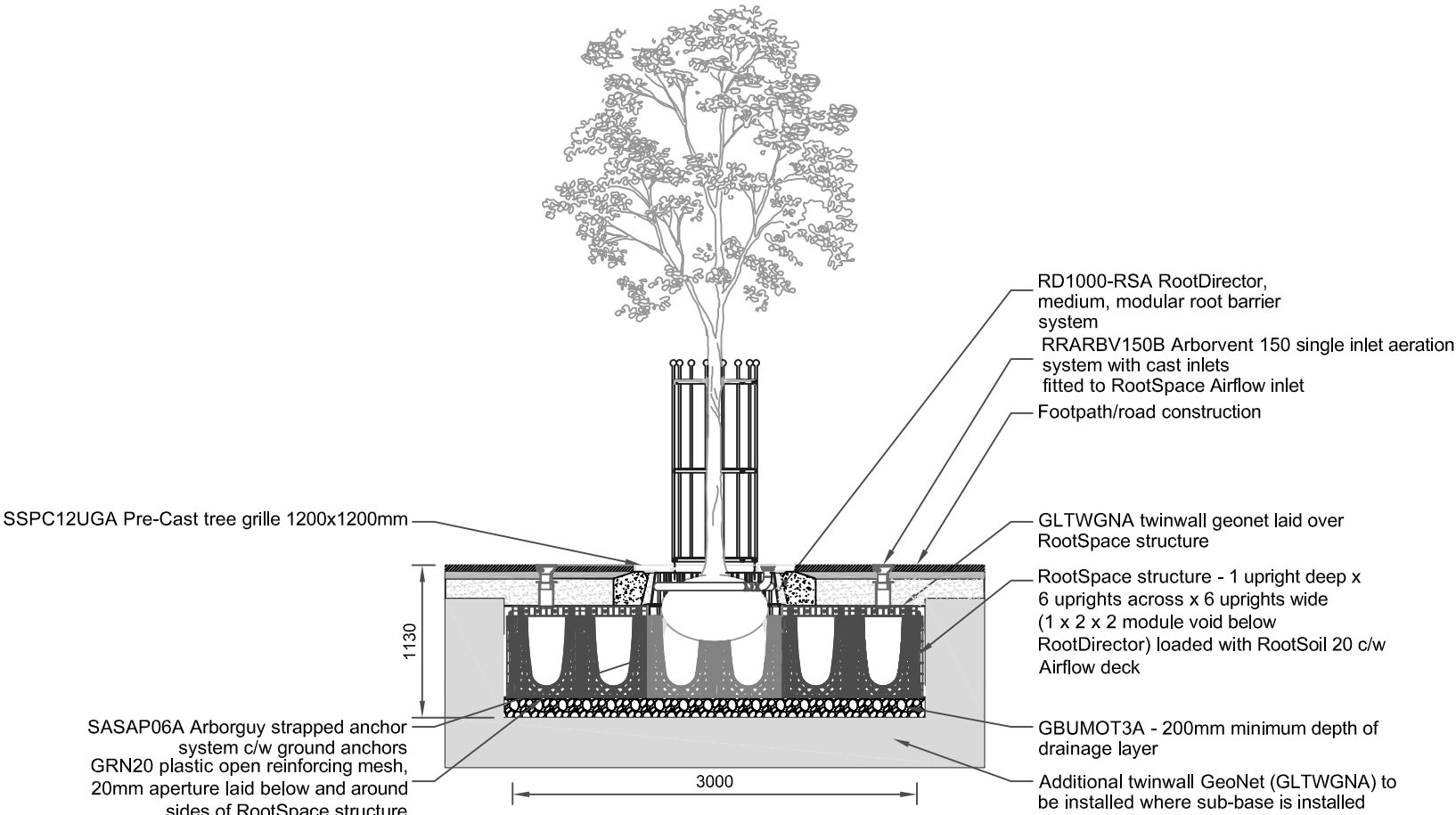
SECTION A-A
